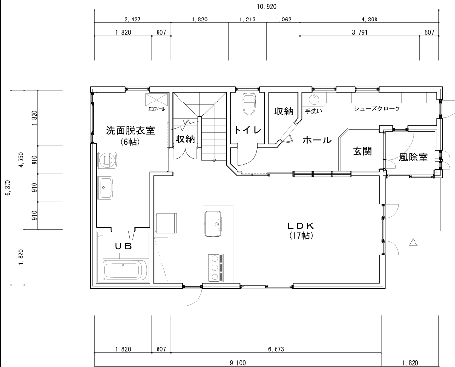
1階 平面図
