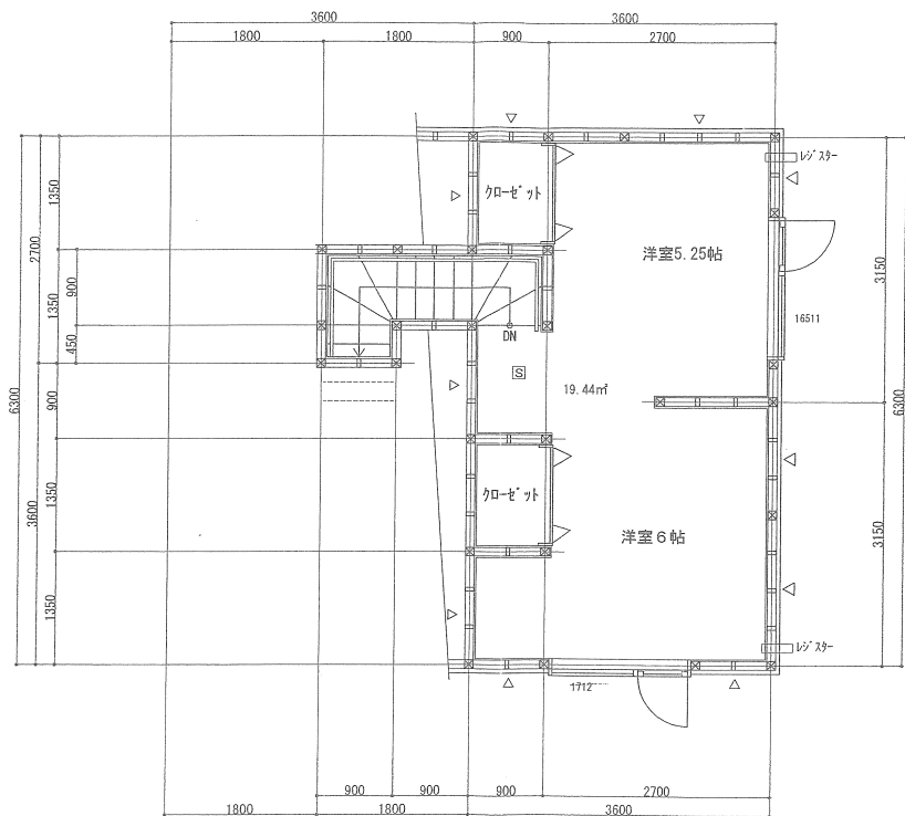
2階平面図 S=1/100
