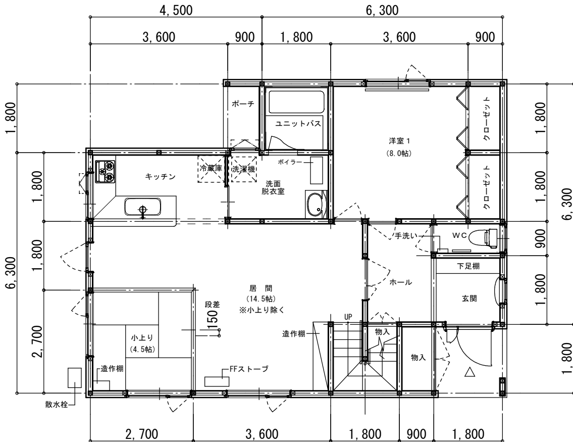
1階平面図
