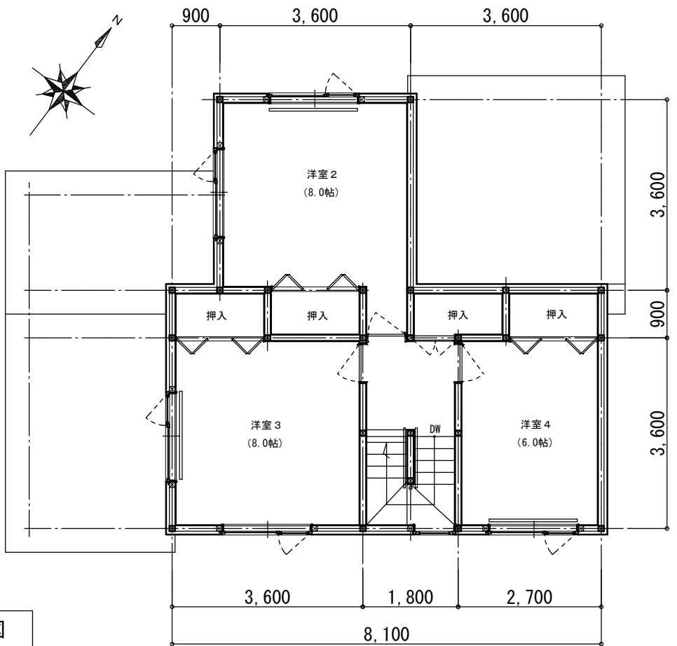
2階平面図
